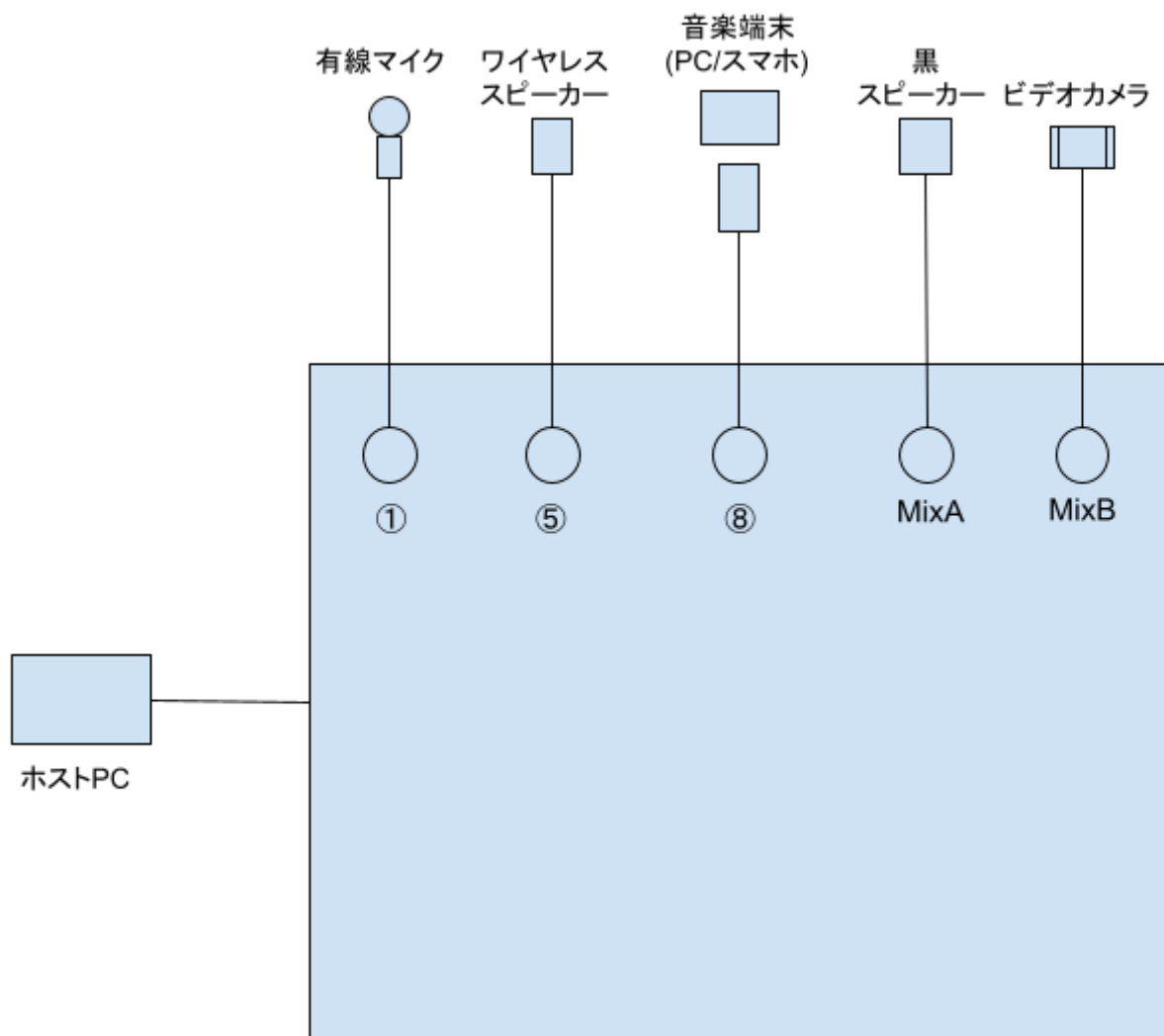
サウンドミキサー機材接続図
